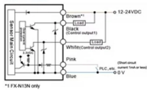
2 Output NPN FX-N13N / N14N
